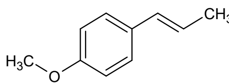
Anetol (no óleo de anis)
