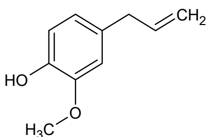
Eugenol (no óleo de cravos)
