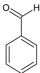
Benzaldeído (no óleo de amêndoas)
