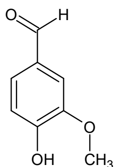
Vanilina (no óleo de baunilha)
