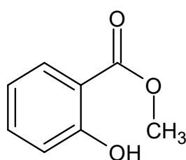
Salicilato de metila (no óleo de gaultéria)
