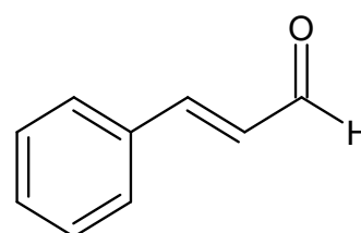
Cinamaldeído (no óleo de canela)
